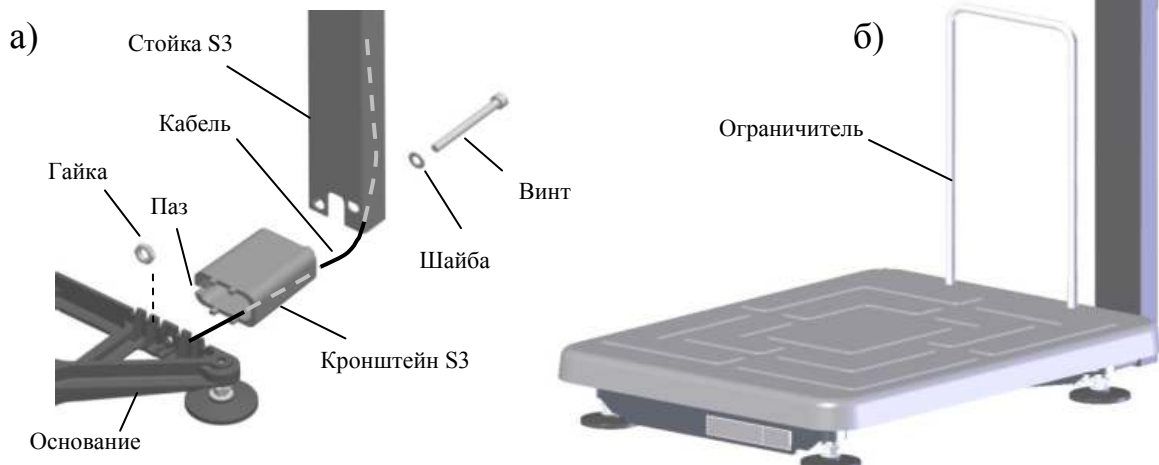
Рис. 5.2 – Крепление прямоугольной стойки к модулю ТВ-S_
